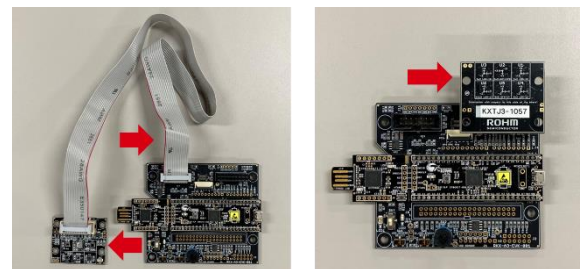
リボンケーブル接続 直接接続 Figure 2. KXTJ3-1057-EVK-001 の接続
