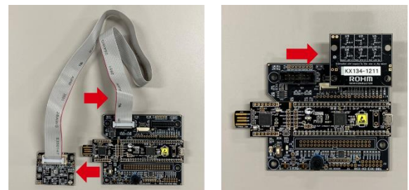
リボンケーブル接続 直接接続 Figure 2. KX134-1211-EVK-001 の接続
