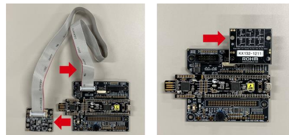
リボンケーブル接続 直接接続 Figure 2. KX132-1211-EVK-001 の接続
